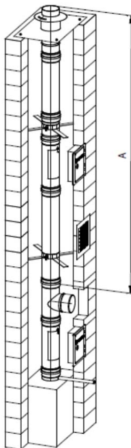
Skica: Max. dovoljena (A) višina dimnika
